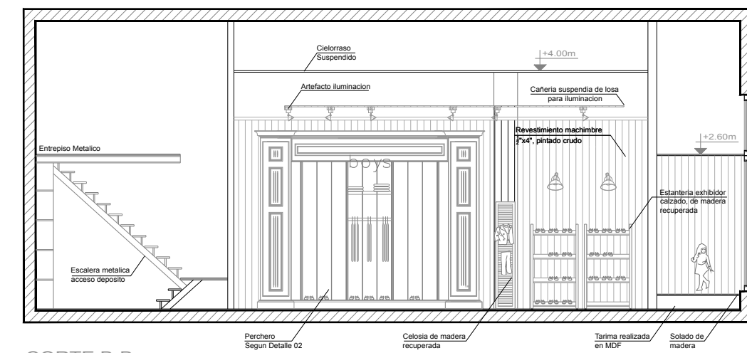
CORTE B-B
