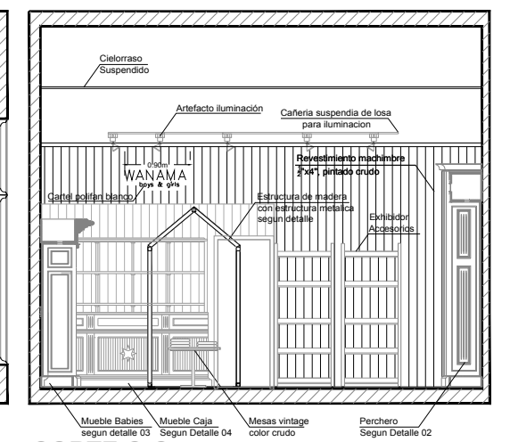
CORTE C-C
